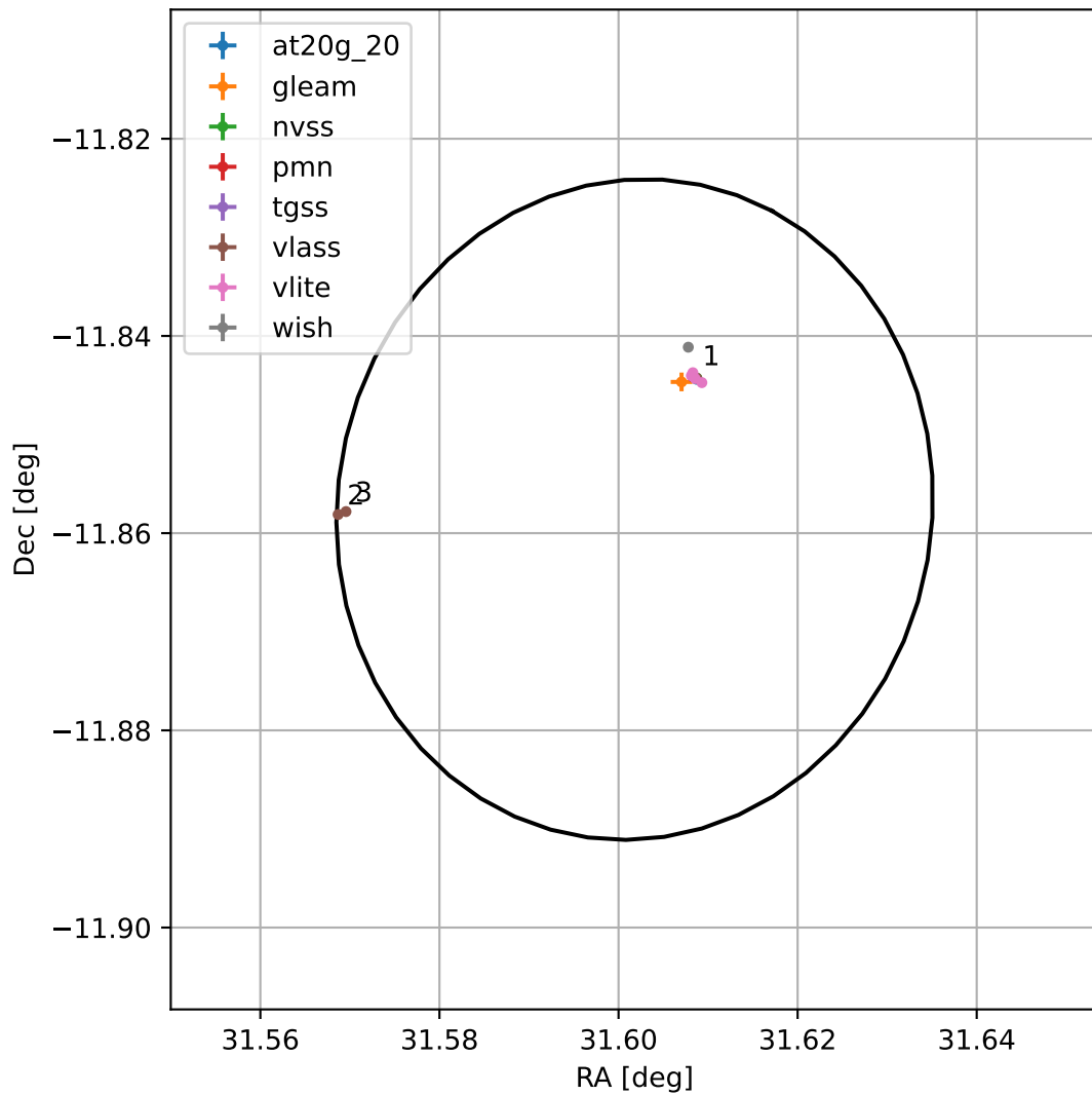
4FGL J0206.4-1151
