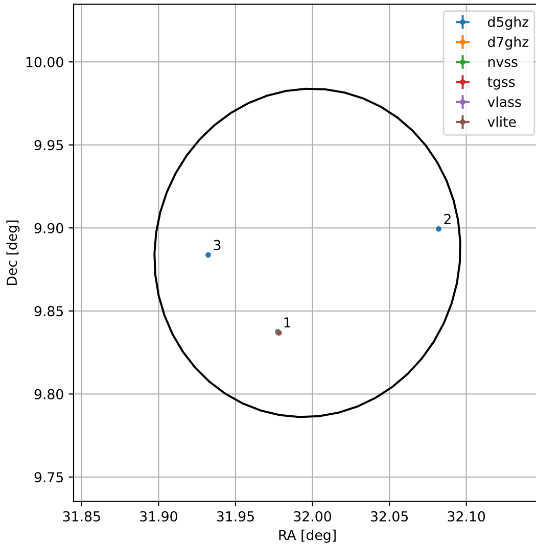
4FGL J0207.9+0953
