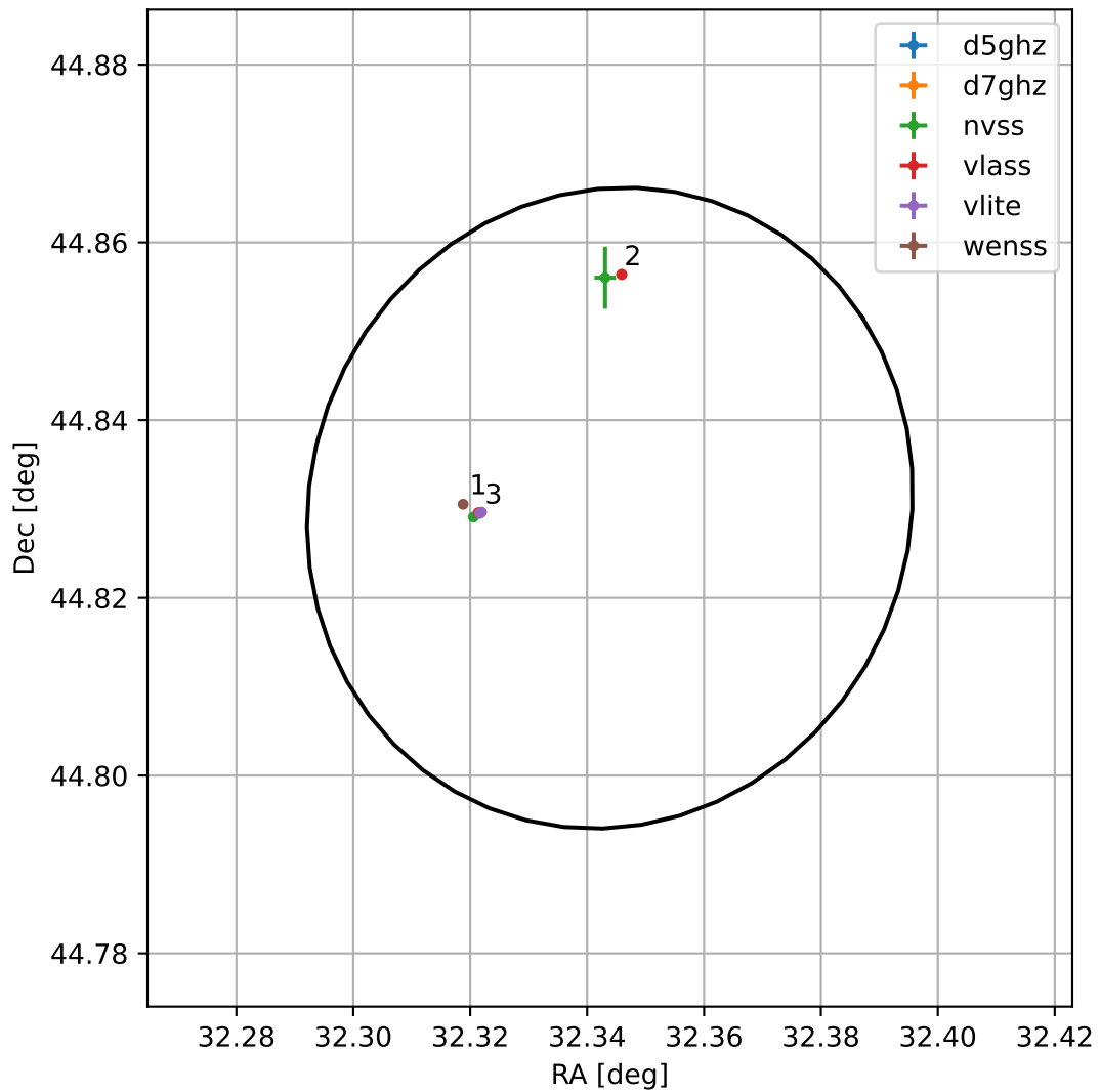
4FGL J0209.3+4449
