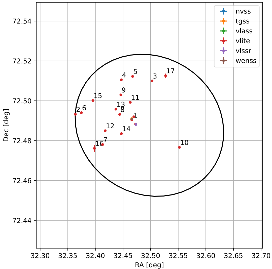
4FGL J0209.9+7229
