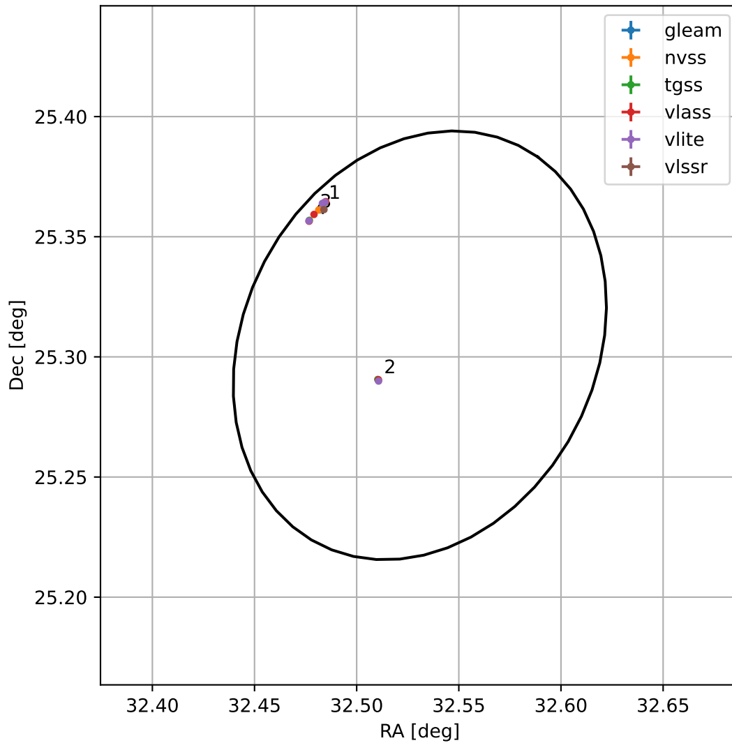
4FGL J0210.1+2518
