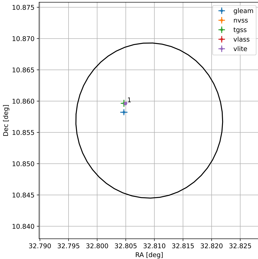
4FGL J0211.2+1051
