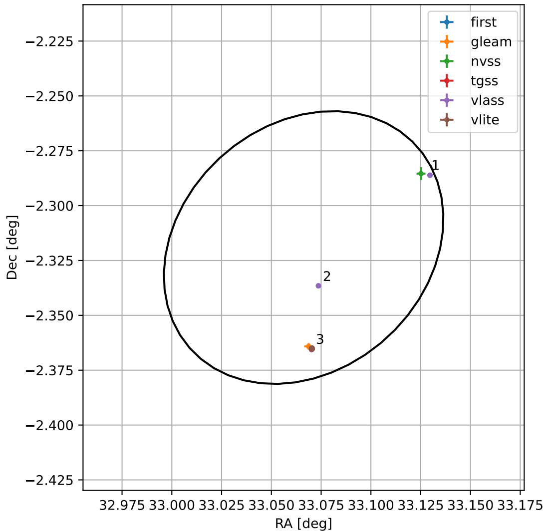
4FGL J0212.2-0219
