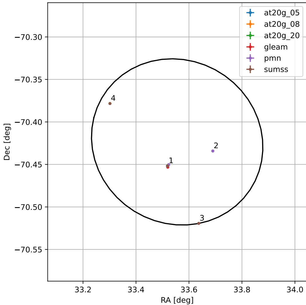
4FGL J0214.2-7025
