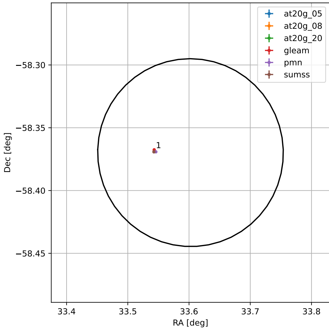
4FGL J0214.4-5822
