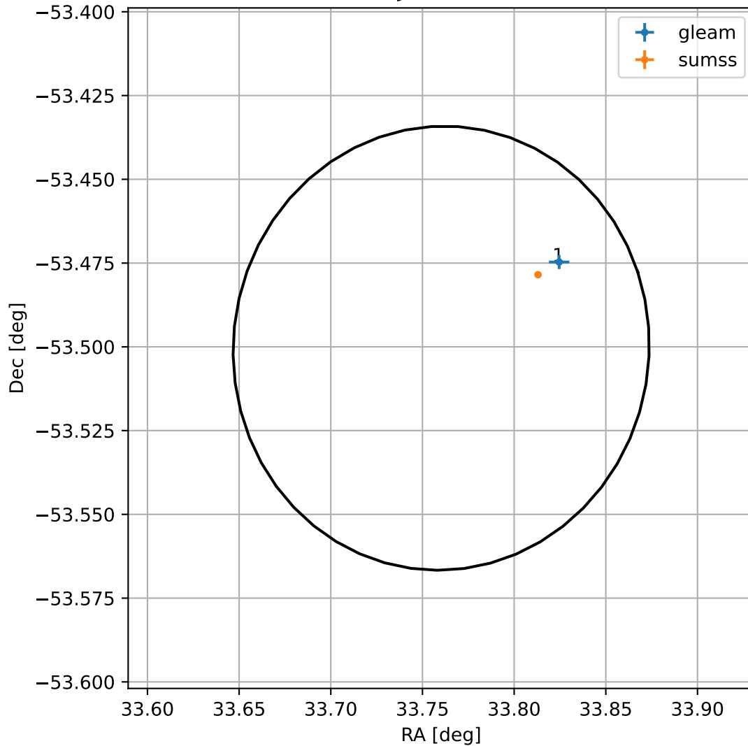
4FGL J0215.0-5330
