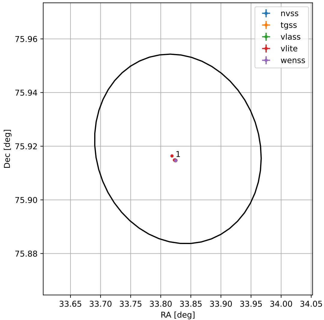
4FGL J0215.3+7555
