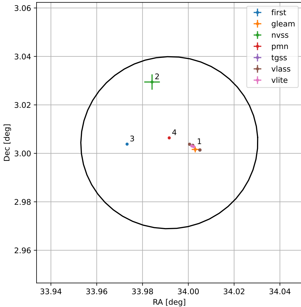
4FGL J0215.9+0300
