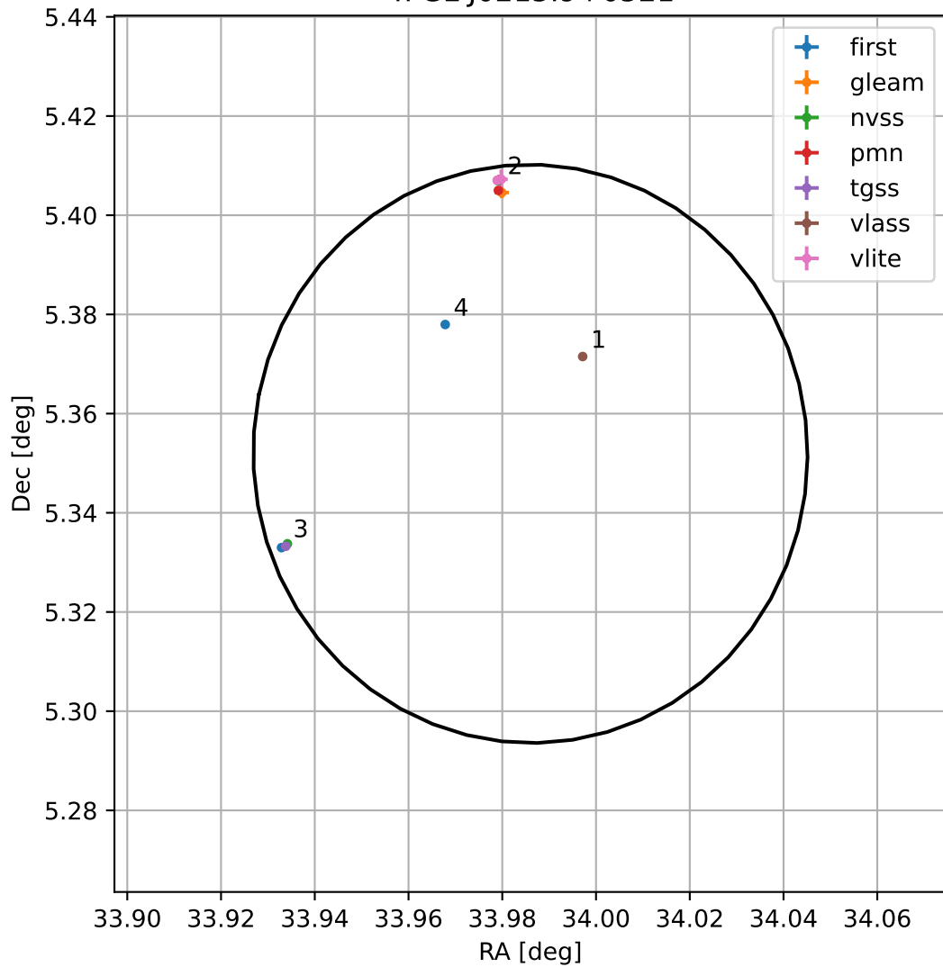
4FGL J0215.9+0521
