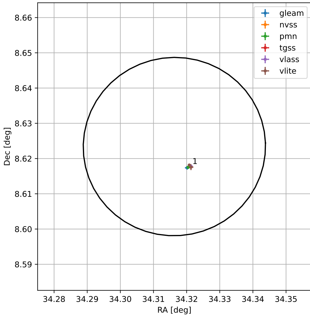
4FGL J0217.2+0837
