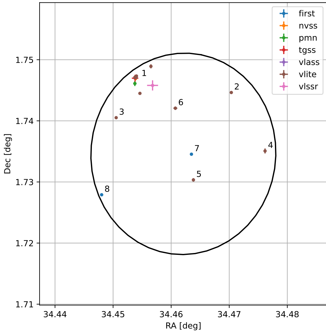
4FGL J0217.8+0144
