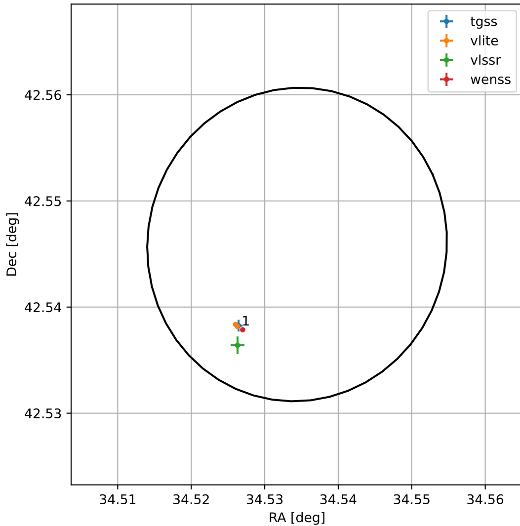
4FGL J0218.1+4232
