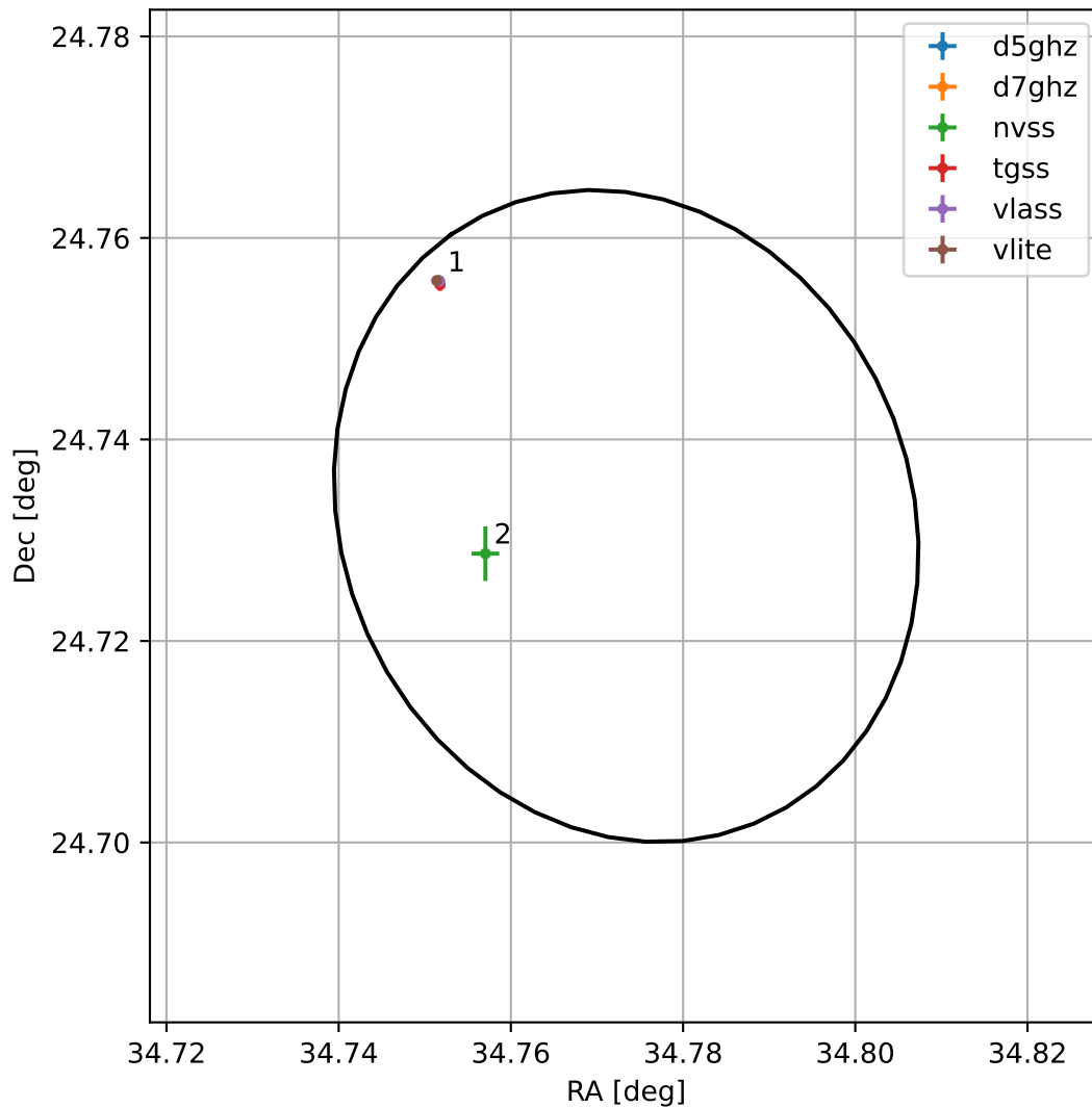
4FGL J0219.0+2443
