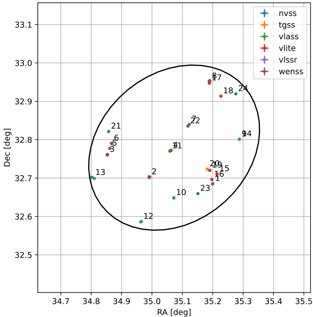
4FGL J0220.2+3246
