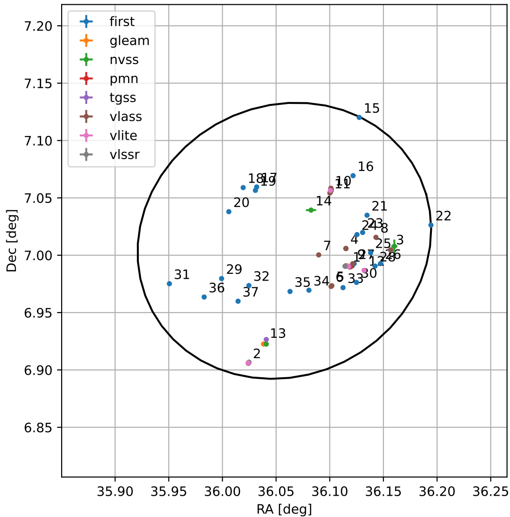
4FGL J0224.2+0700
