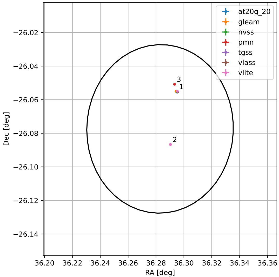
4FGL J0225.1-2604
