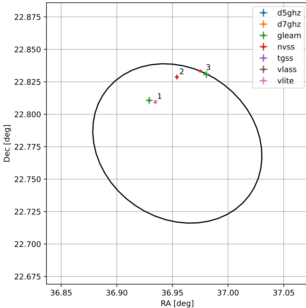
4FGL J0227.8+2246
