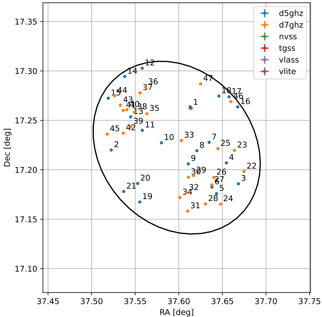
4FGL J0230.3+1713
