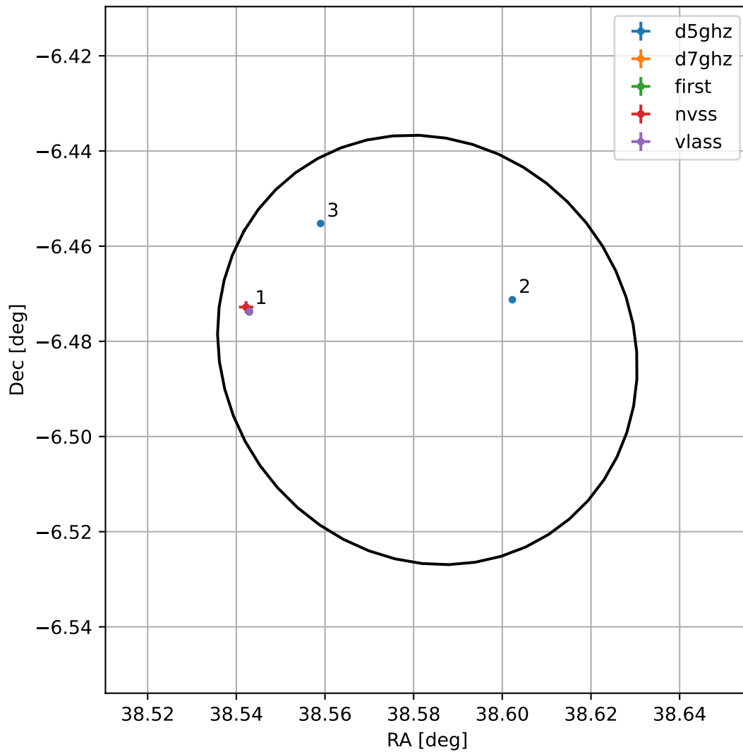
4FGL J0234.3-0628
