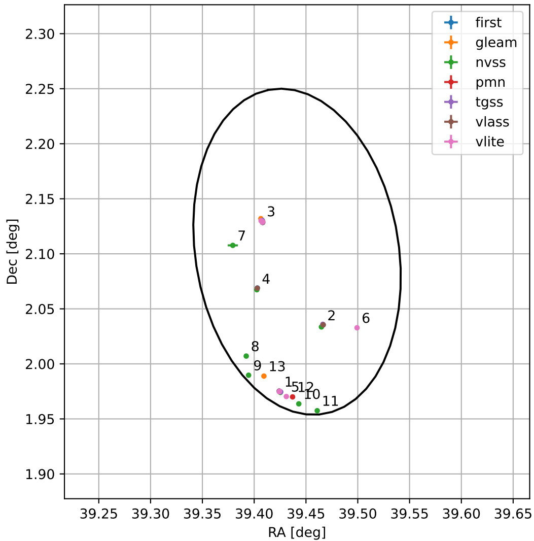
4FGL J0237.7+0206
