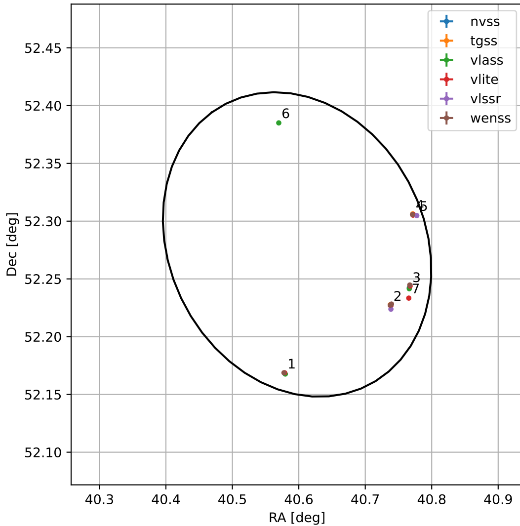
4FGL J0242.3+5216
