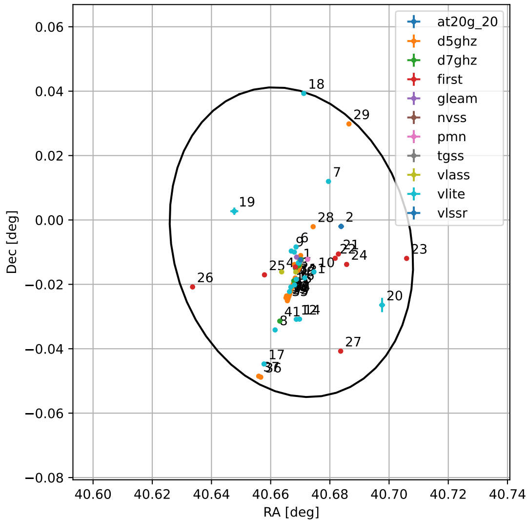
4FGL J0242.6-0000
