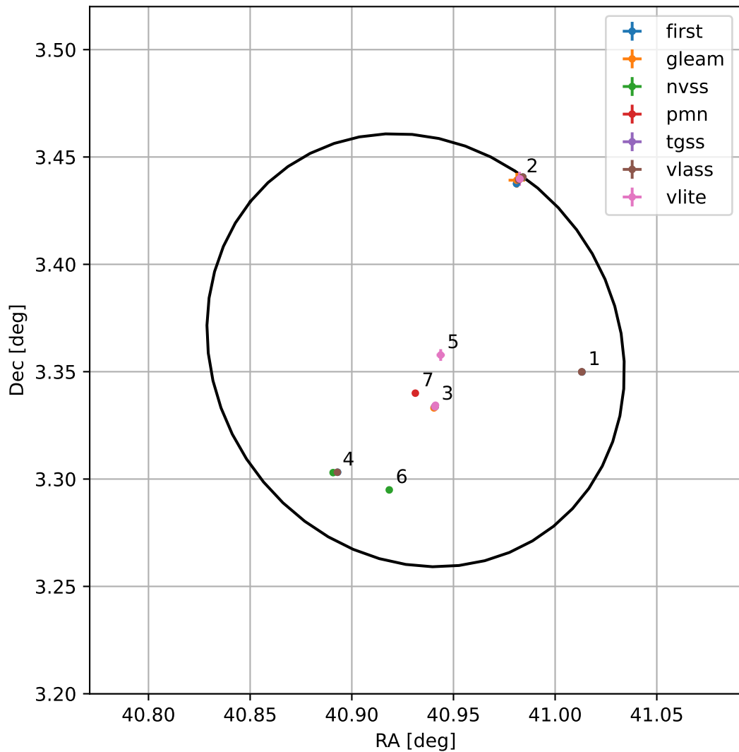
4FGL J0243.7+0321
