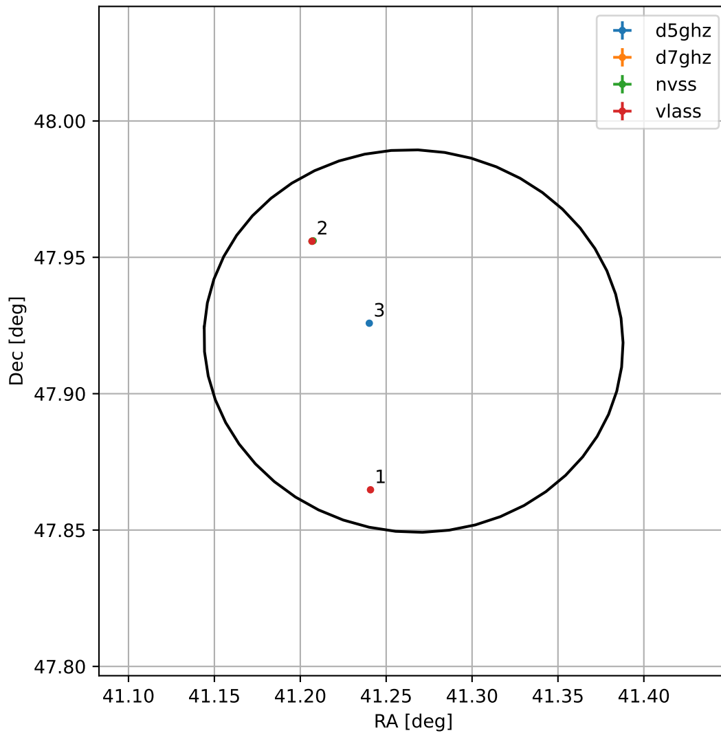
4FGL J0245.0+4755
