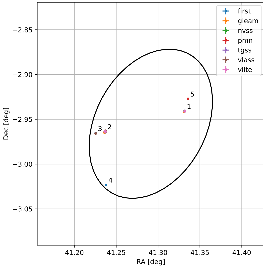
4FGL J0245.1-0257
