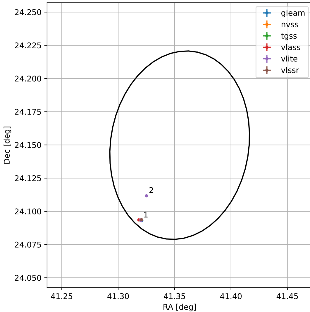
4FGL J0245.4+2408
