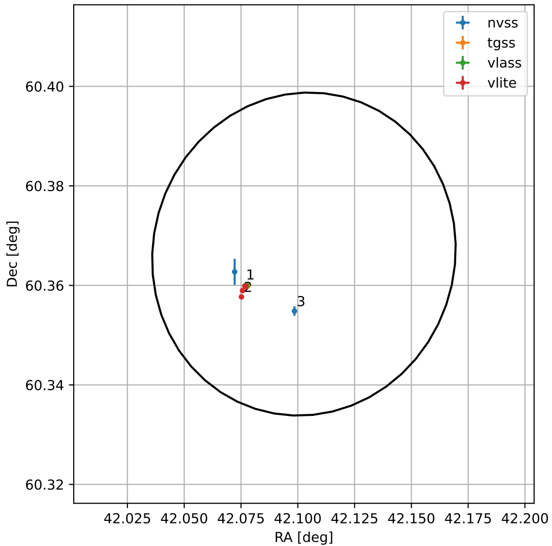
4FGL J0248.4+6021
