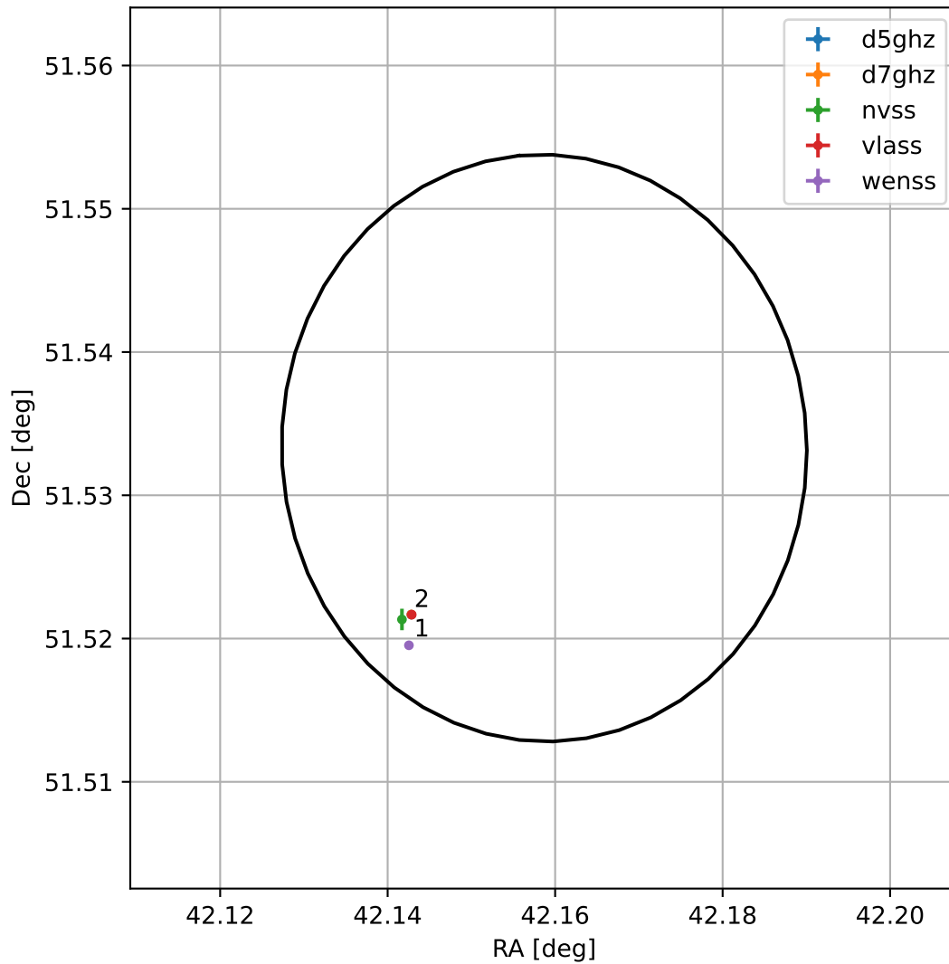
4FGL J0248.6+5131
