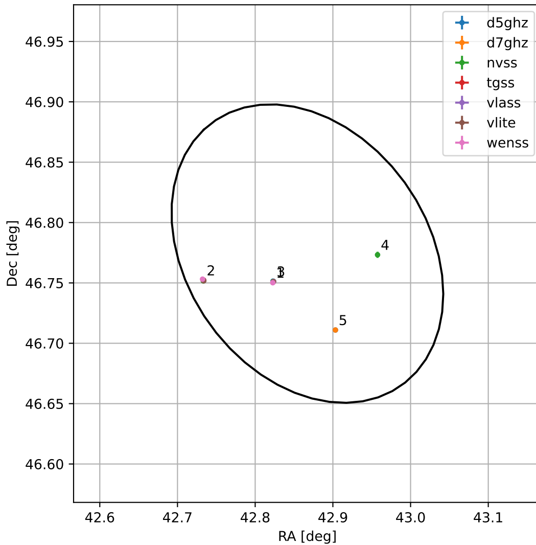
4FGL J0251.4+4646
