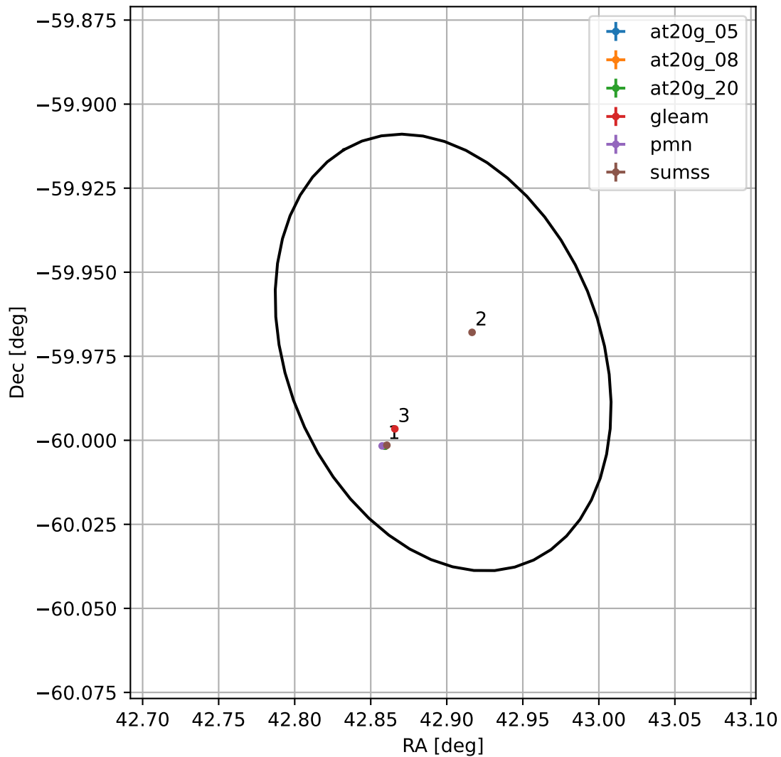
4FGL J0251.5-5958
