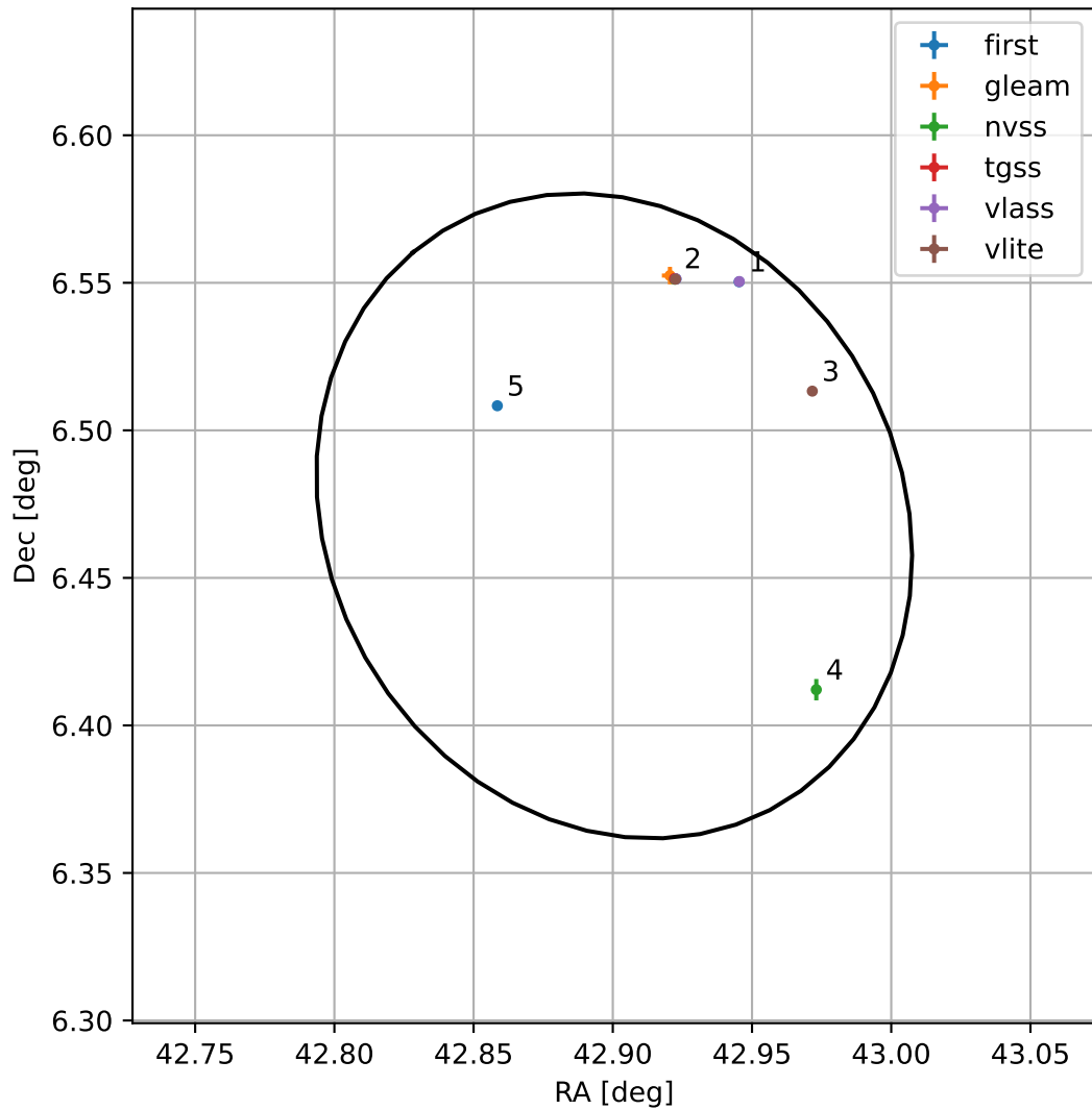
4FGL J0251.6+0628
