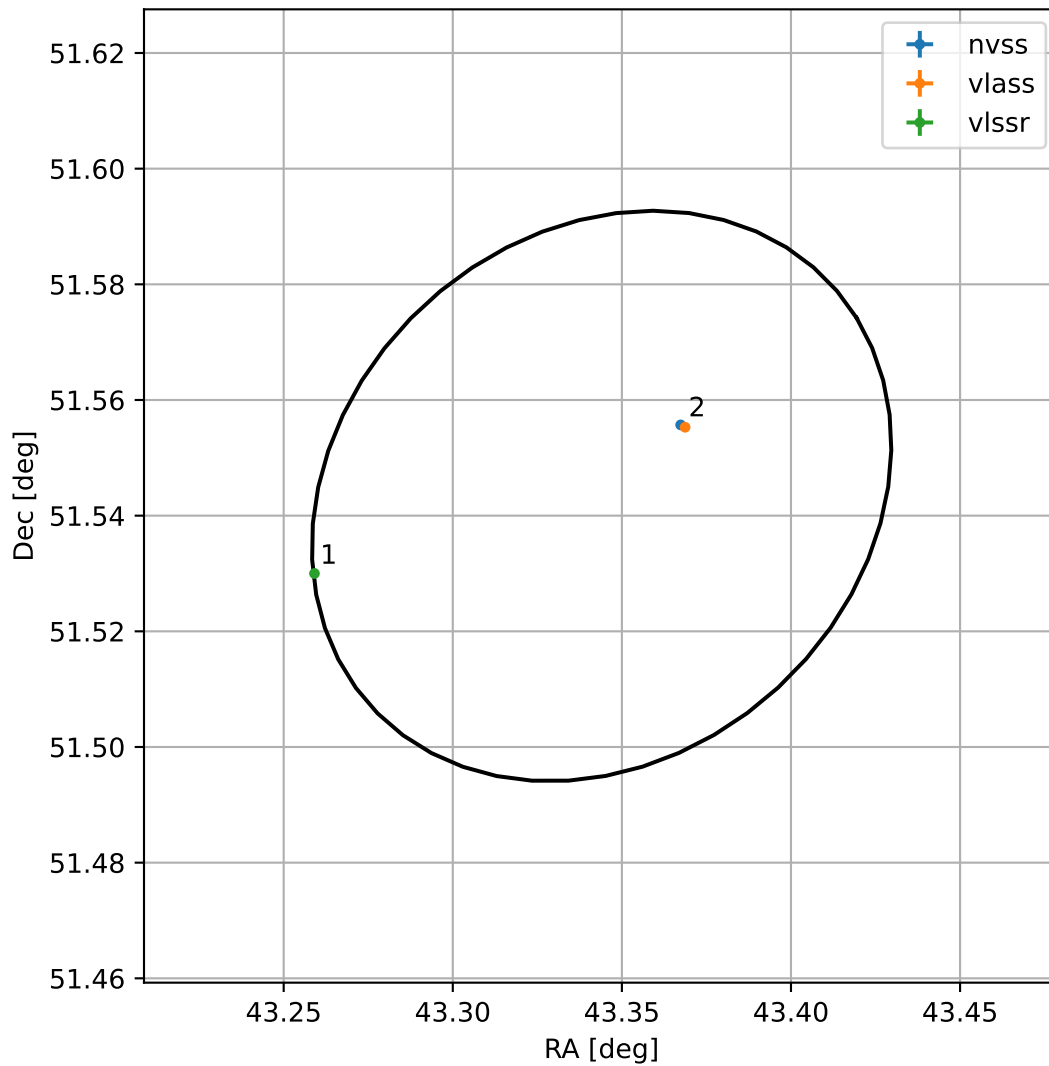
4FGL J0253.3+5132
