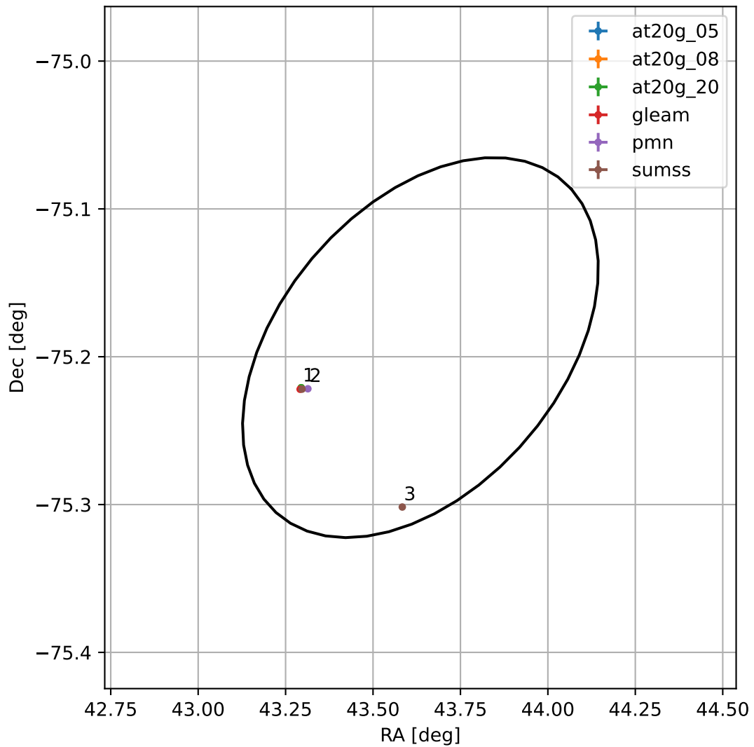
4FGL J0254.5-7511
