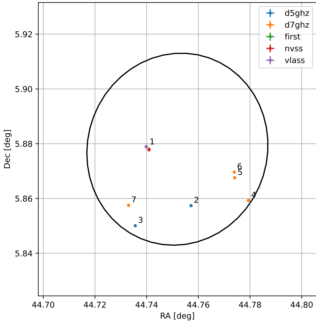
4FGL J0259.0+0552
