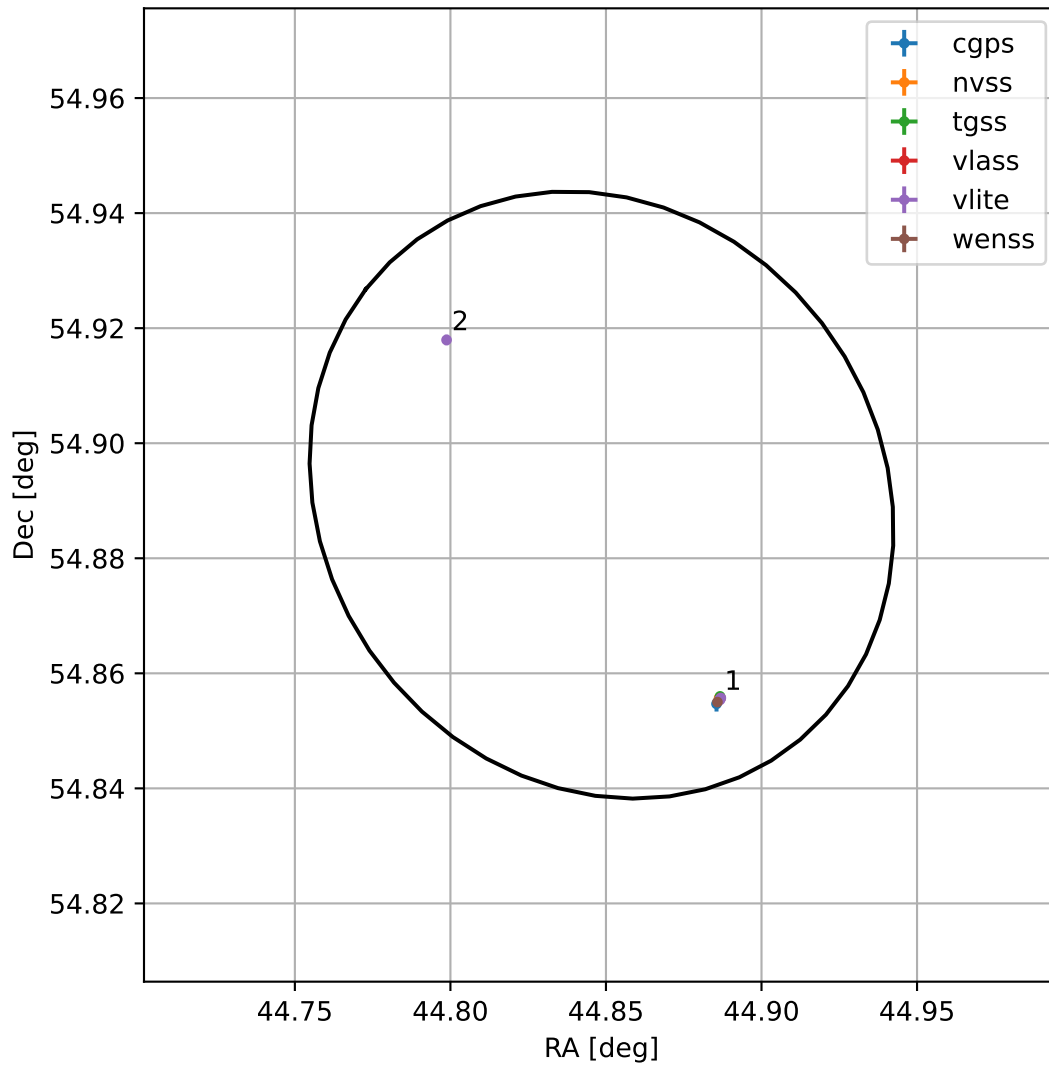
4FGL J0259.3+5453
