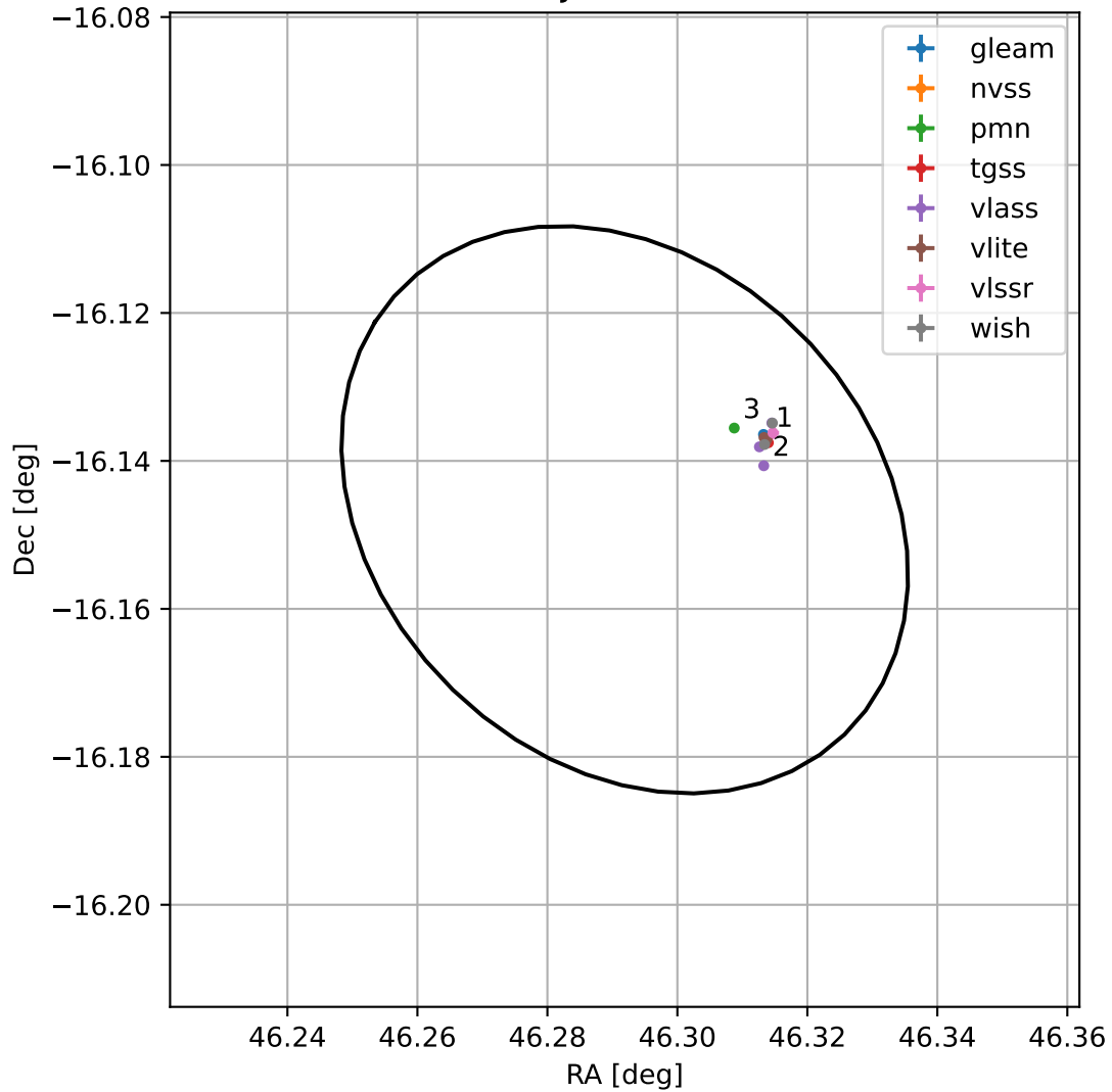
4FGL J0305.1-1608
