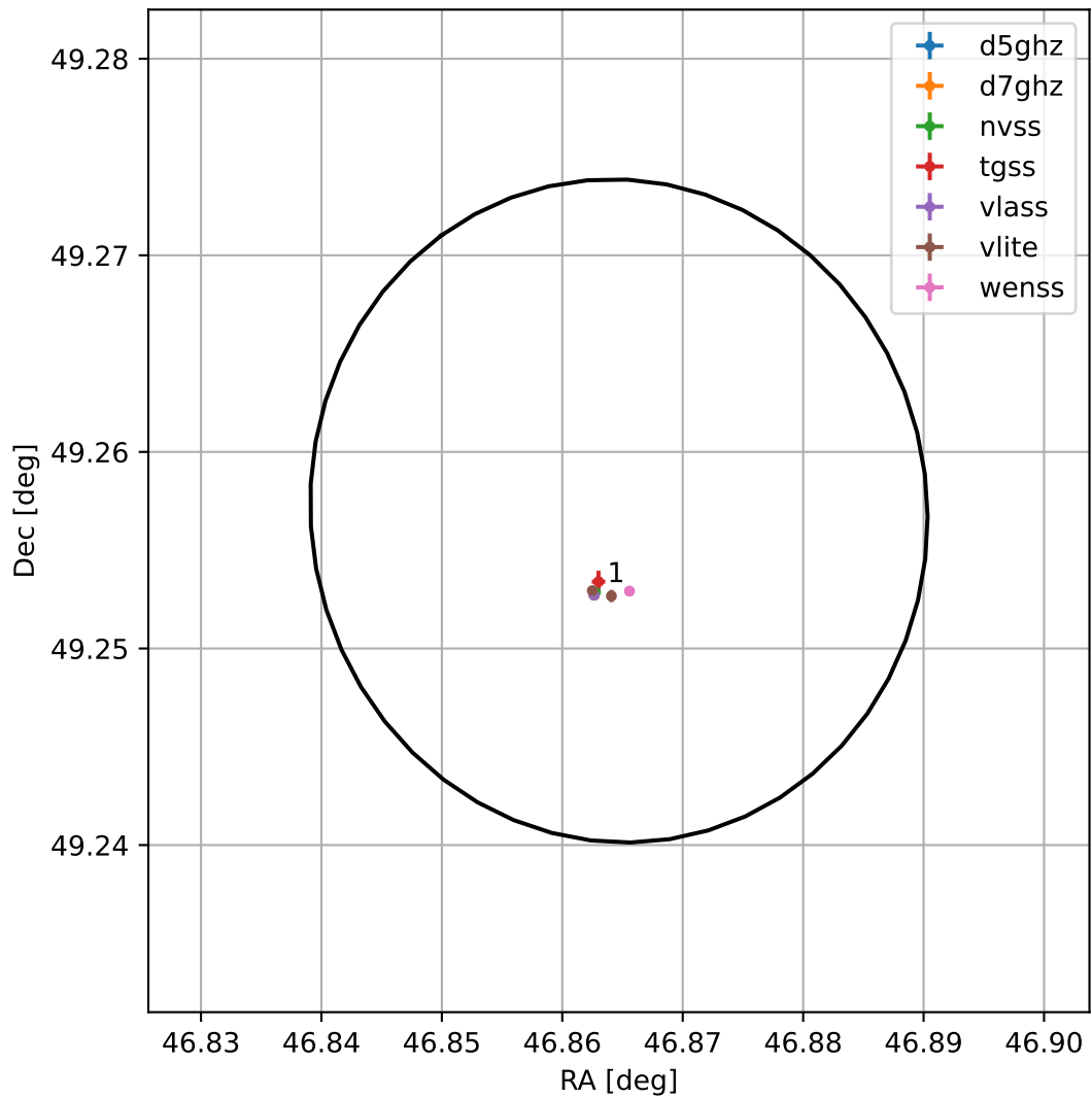
4FGL J0307.4+4915
