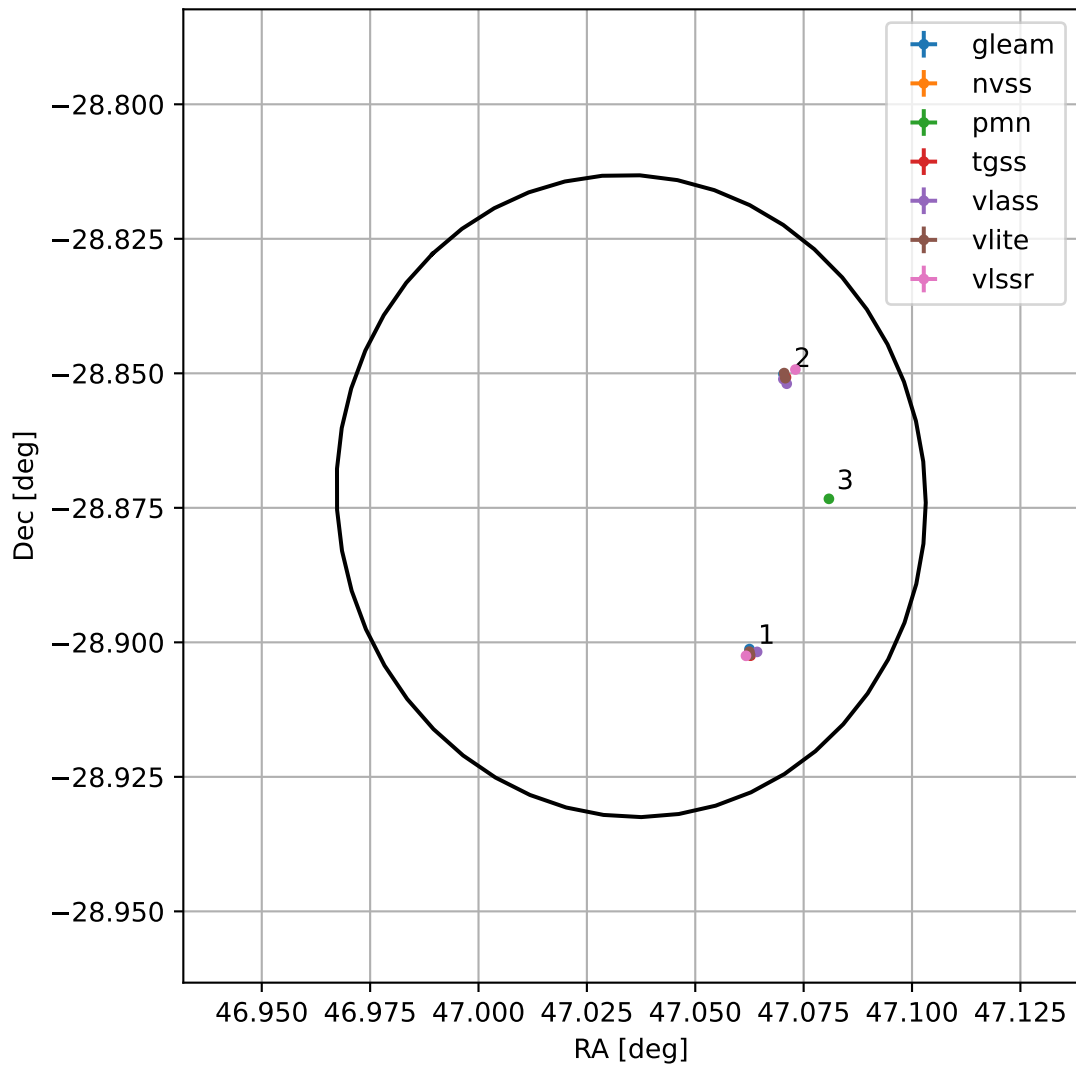
4FGL J0308.1-2852
