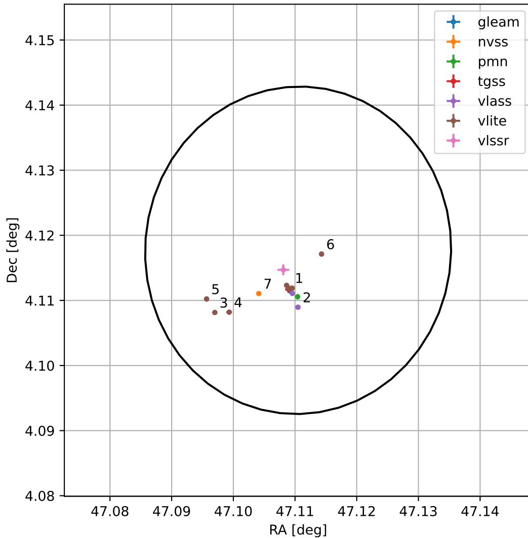
4FGL J0308.4+0407
