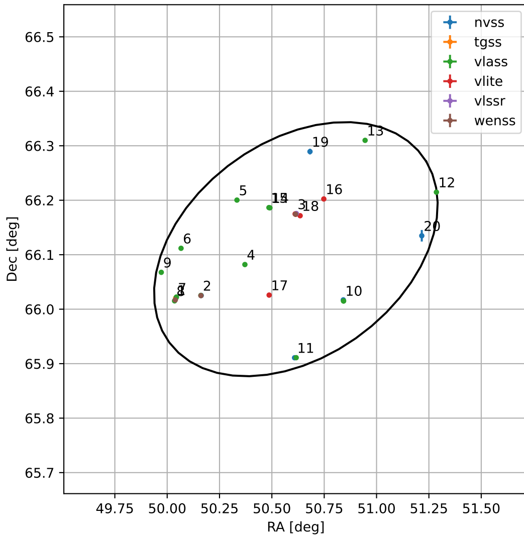
4FGL J0322.4+6606
