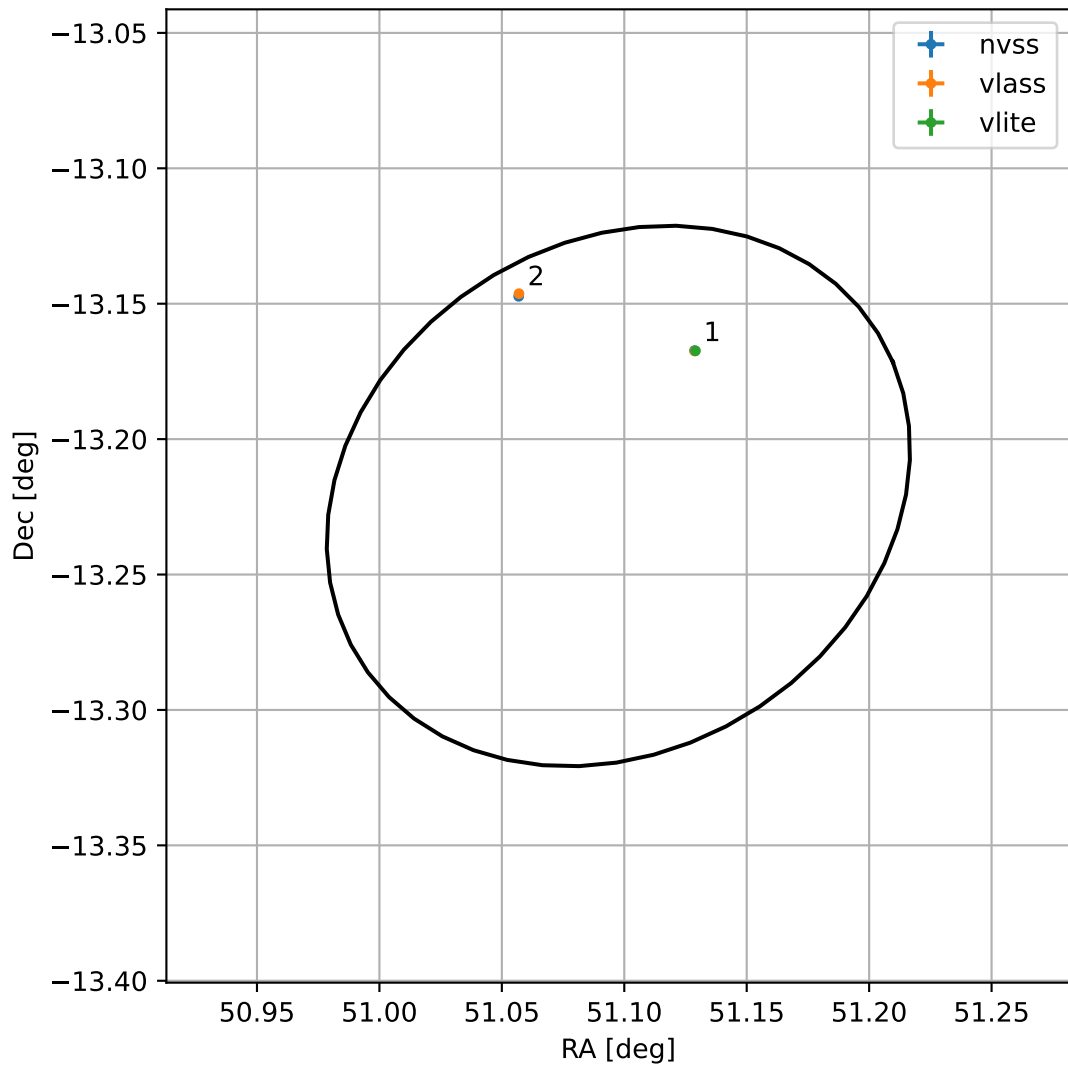
4FGL J0324.3-1313
