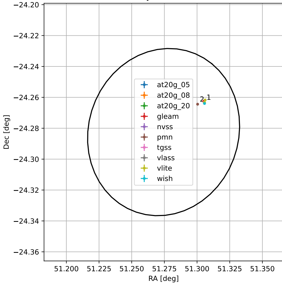
4FGL J0325.0-2416
