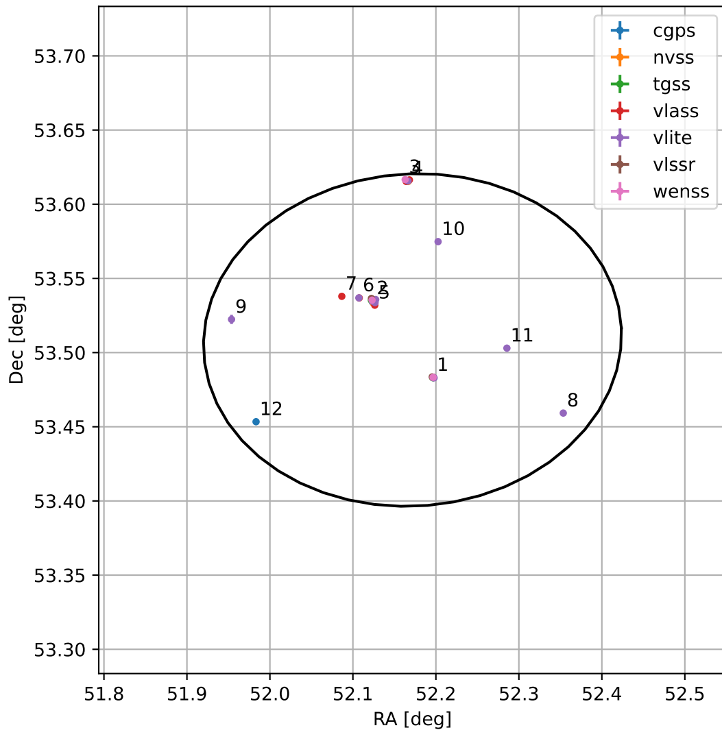
4FGL J0328.6+5330
