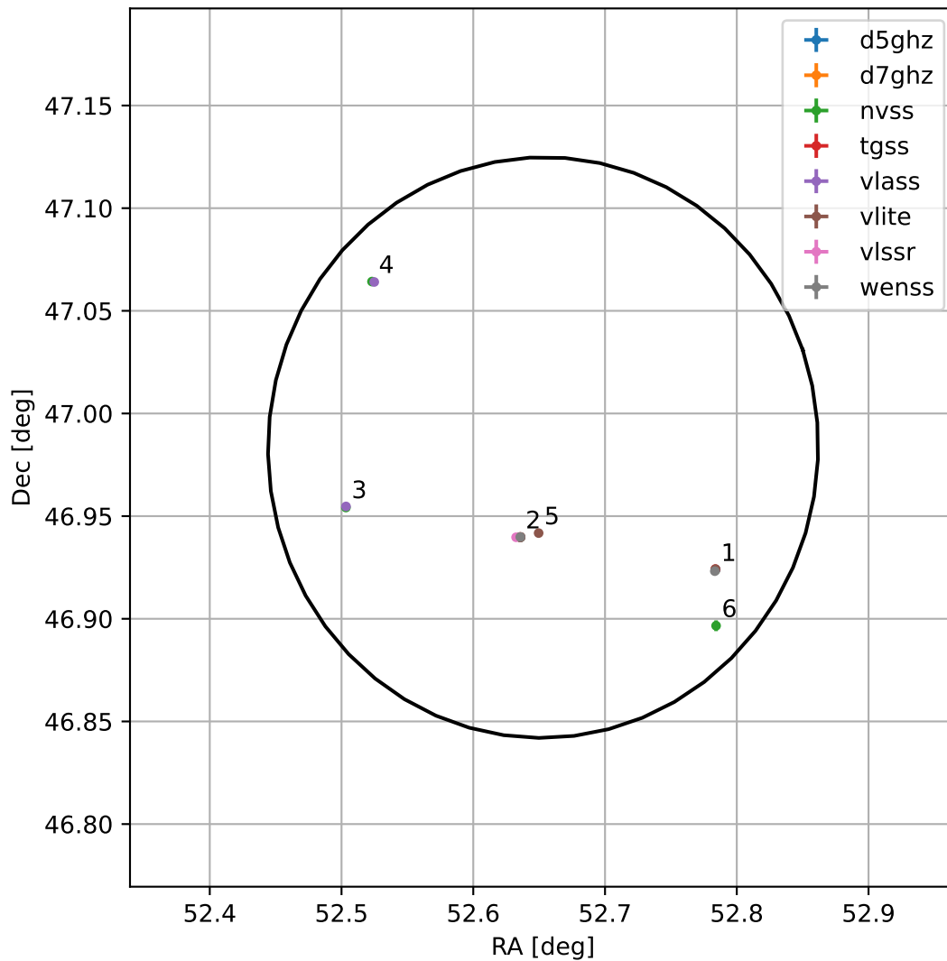
4FGL J0330.6+4659
