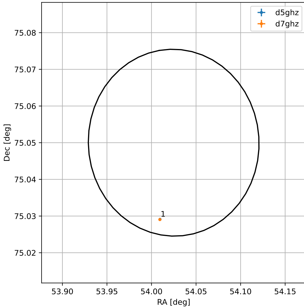
4FGL J0336.0+7502
