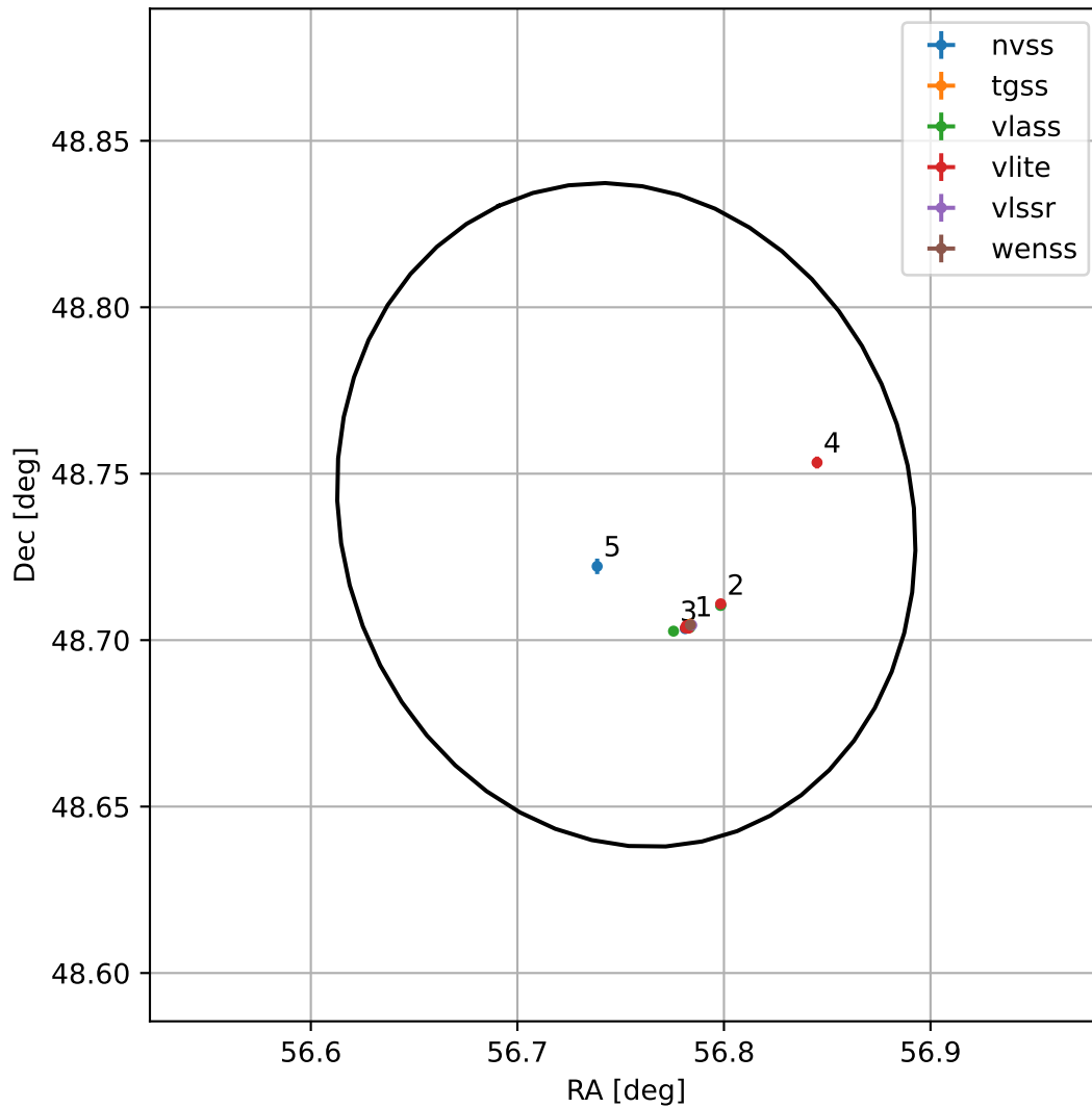
4FGL J0347.0+4844
